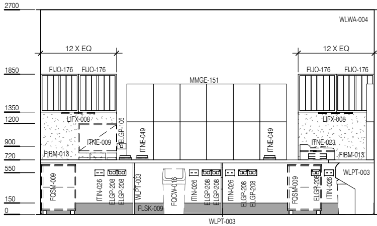
ELEVATION 4
