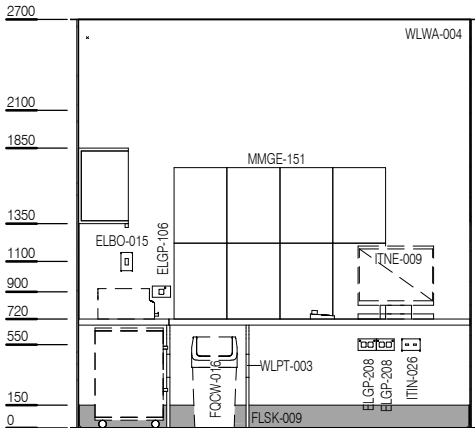
ELEVATION 1
