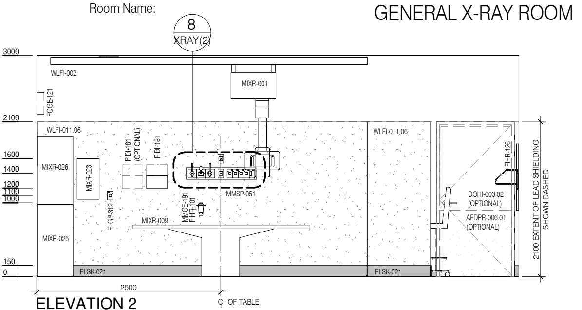
ELEVATION 2
