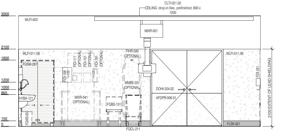
ELEVATION 4
