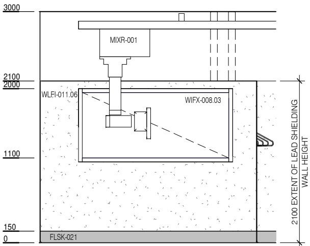
ELEVATION 7
