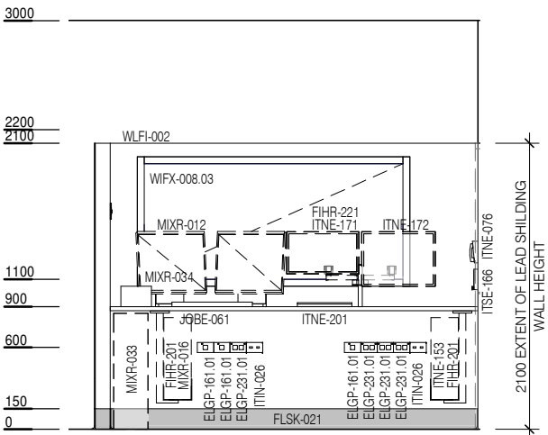
ELEVATION 5
