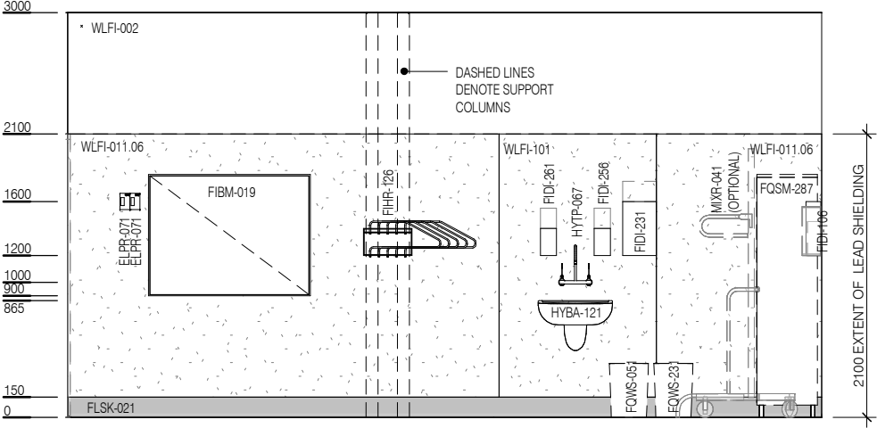
ELEVATION 3
