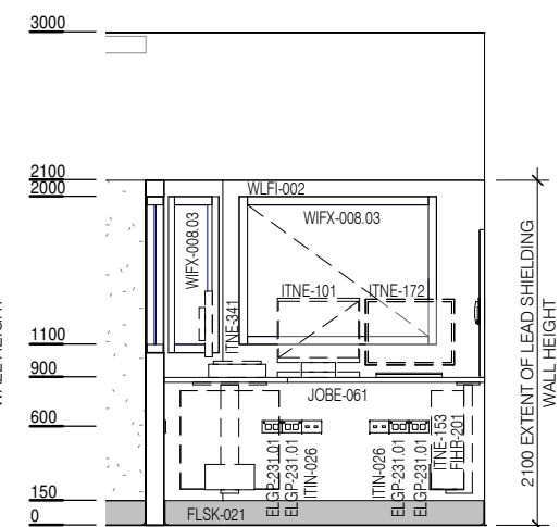
ELEVATION 6
