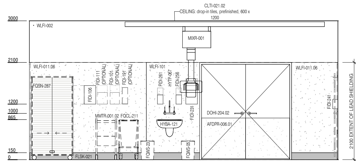
ELEVATION 4
