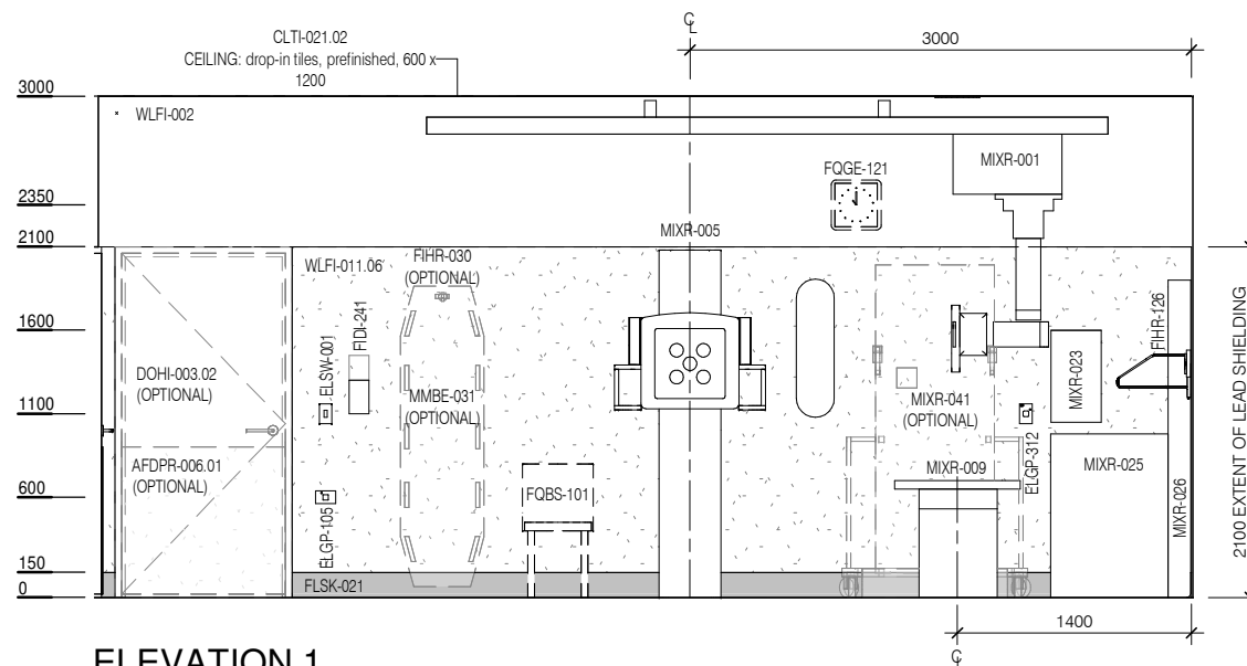
ELEVATION 1
