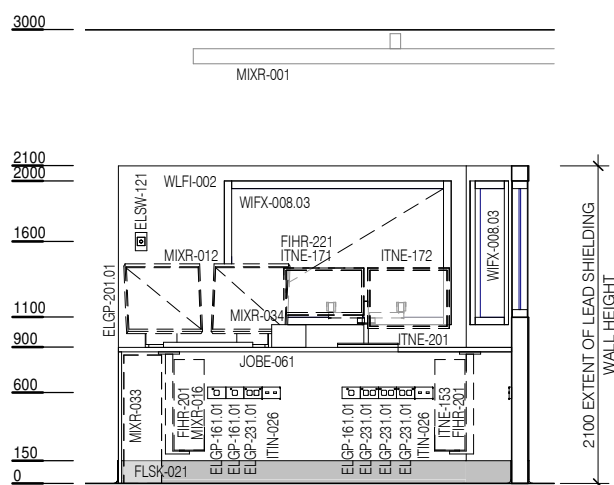
ELEVATION 5
