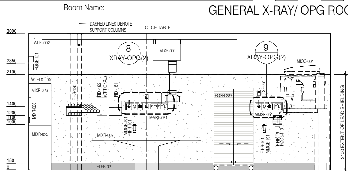
ELEVATION 2
