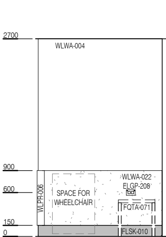
ELEVATION 1
