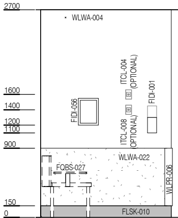
ELEVATION 3
