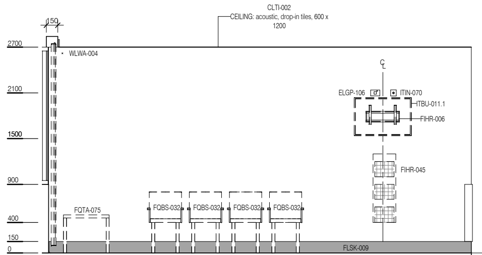
ELEVATION 2
