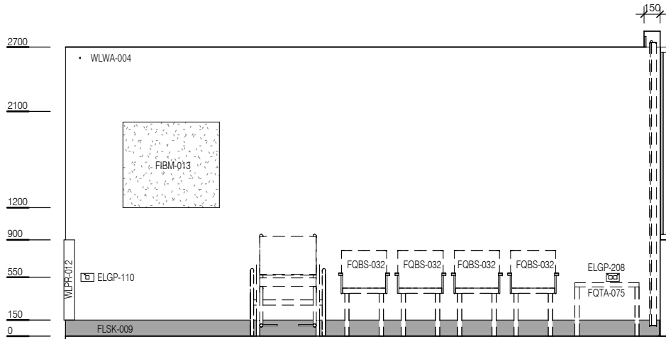
ELEVATION 3
