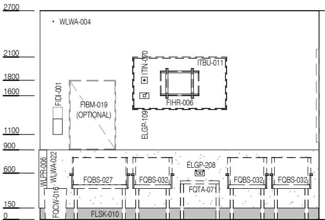
ELEVATION 2
