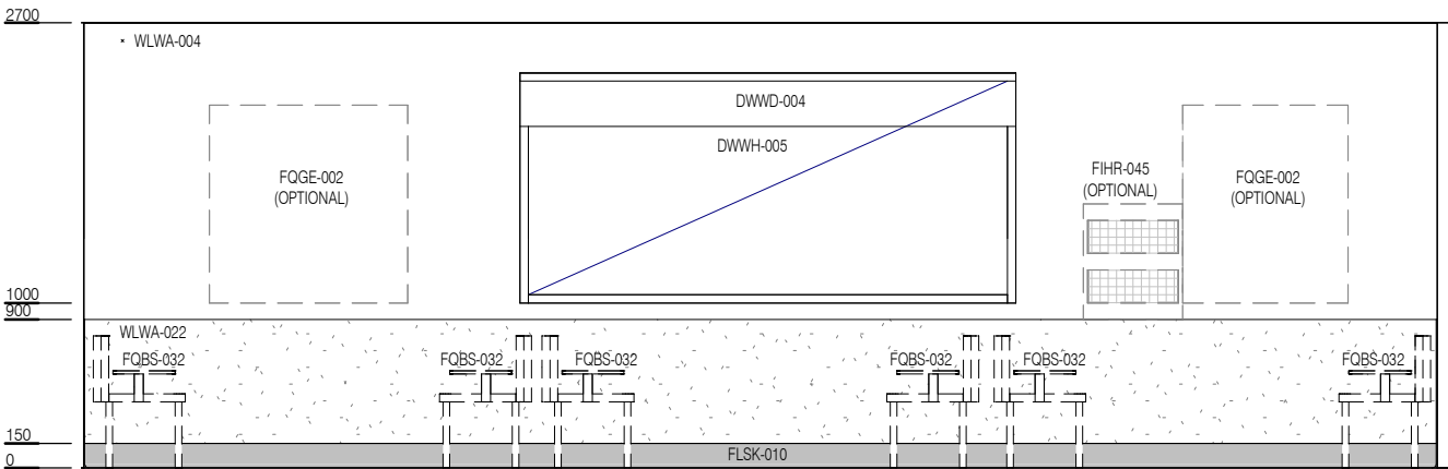
ELEVATION 3
