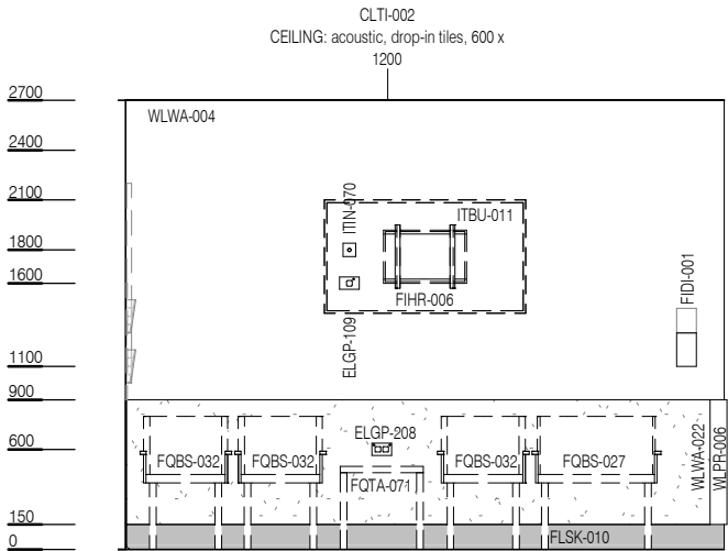
ELEVATION 1
