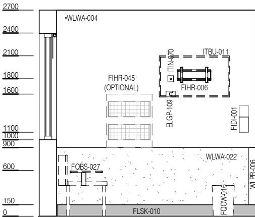
ELEVATION 3
