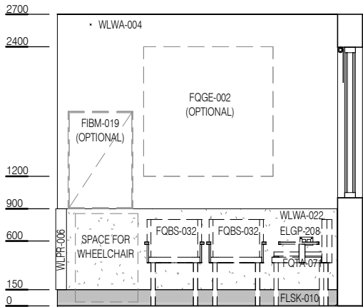
ELEVATION 1
