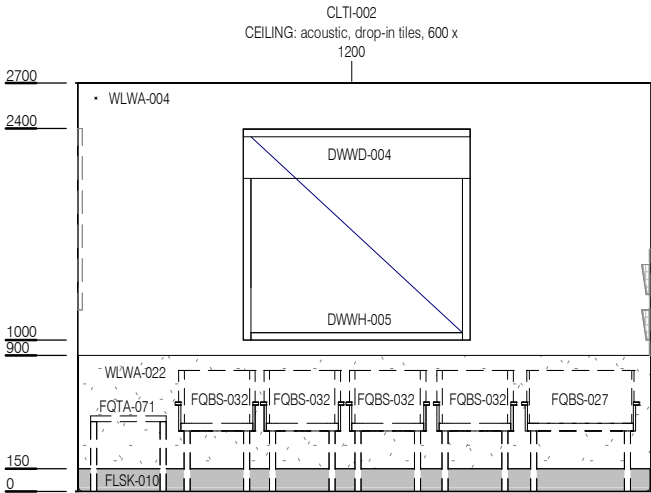
ELEVATION 2
