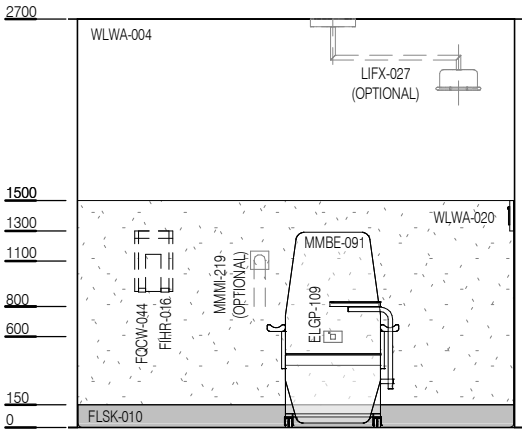
ELEVATION 3
