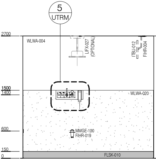
ELEVATION 4
