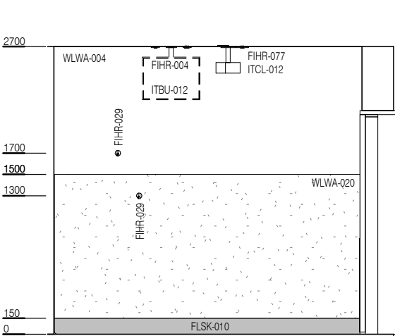
ELEVATION 1
