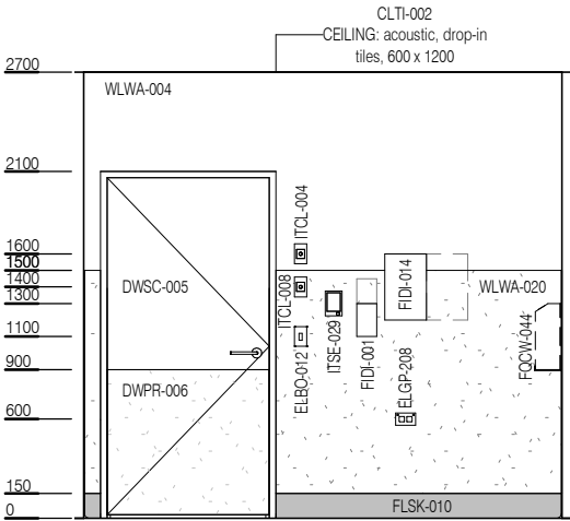
ELEVATION 2
