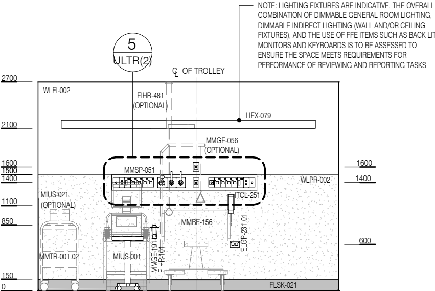
ELEVATION 1
