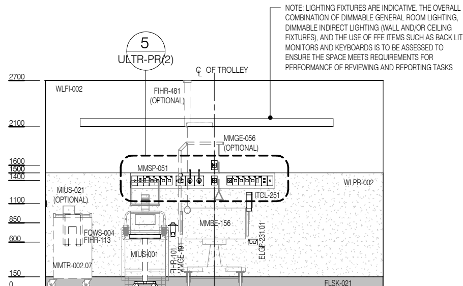
ELEVATION 1
