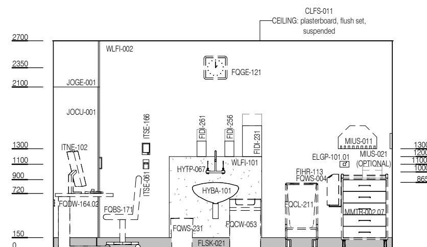
ELEVATION 4
