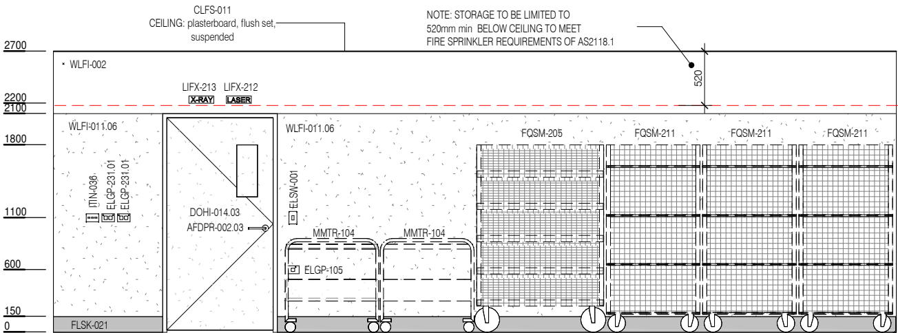
ELEVATION 2
