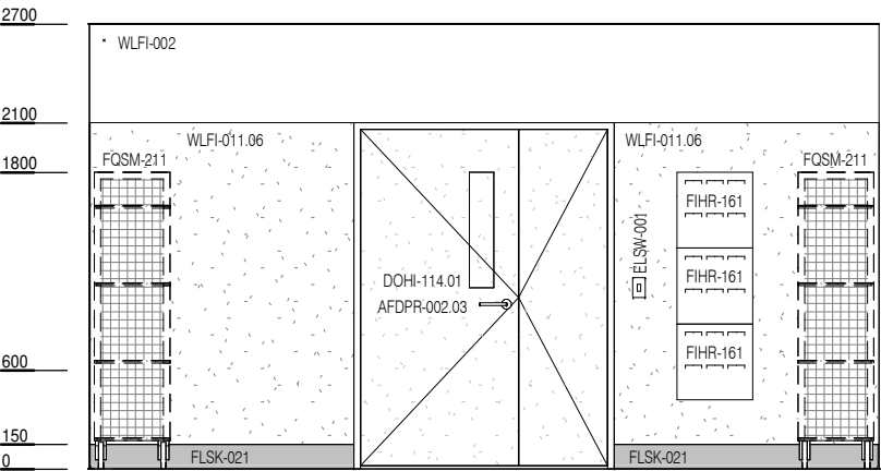
ELEVATION 3
