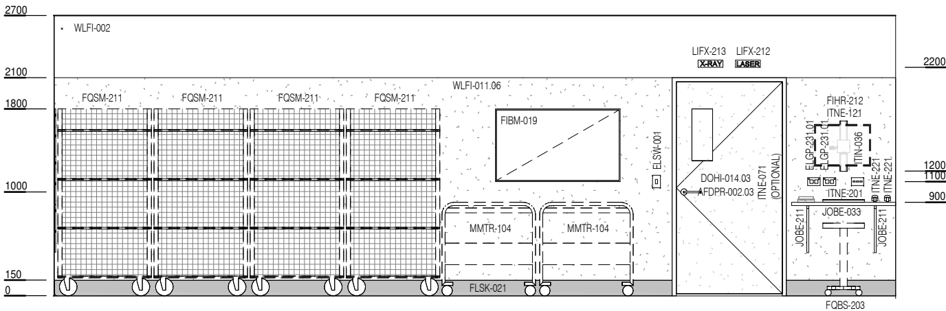
ELEVATION 1
