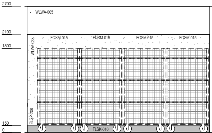
ELEVATION 1
