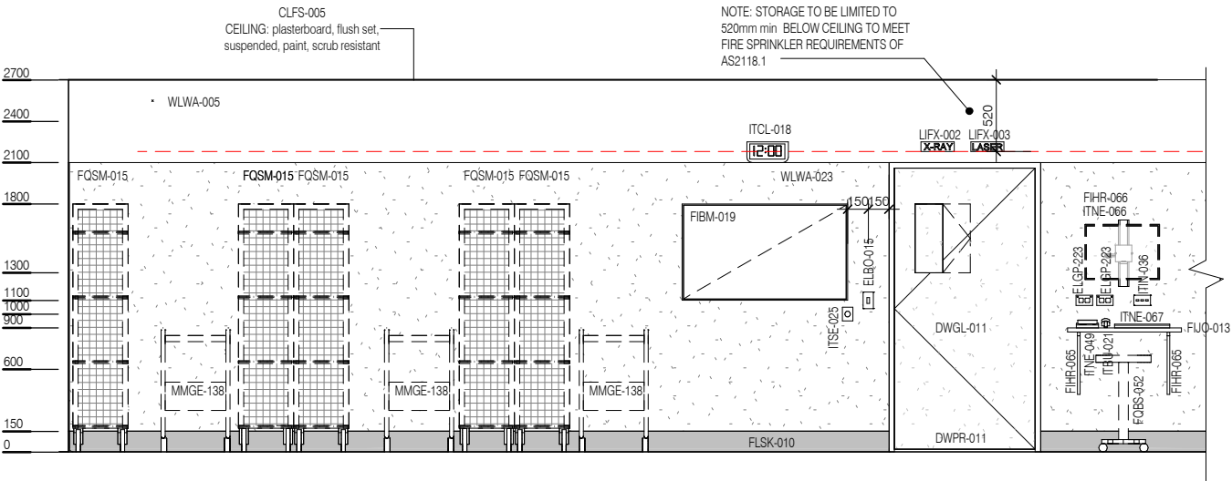
ELEVATION 2
