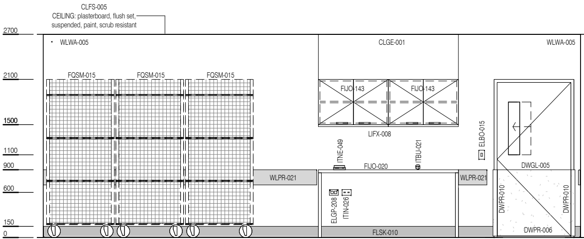
ELEVATION 2
