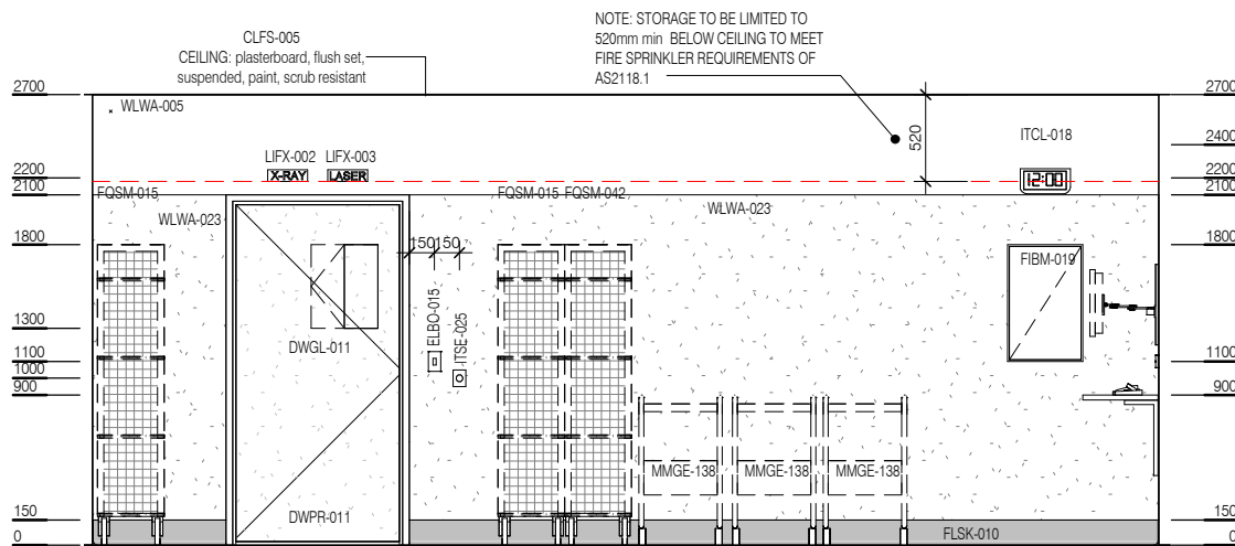
ELEVATION 2
