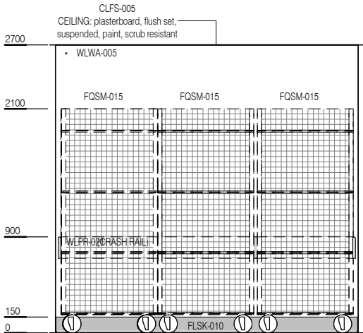
ELEVATION 2
