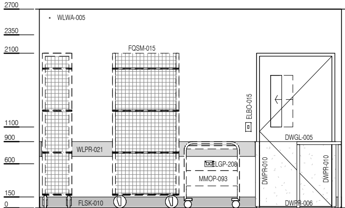
ELEVATION 3
