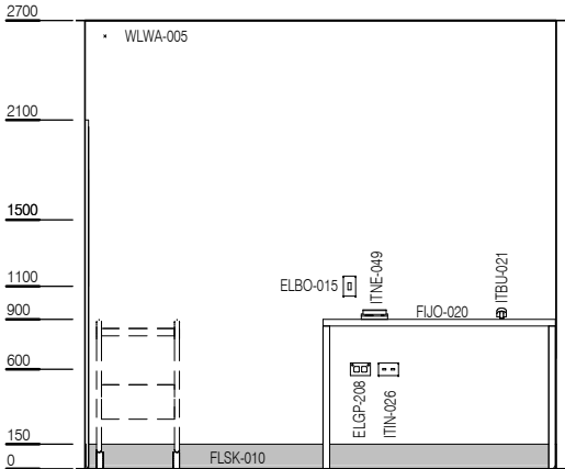
ELEVATION 4
