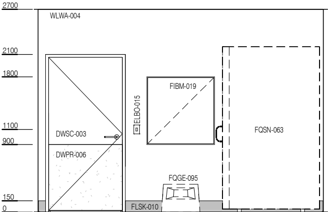
ELEVATION 3
