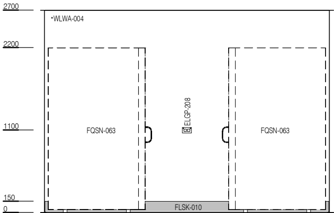
ELEVATION 1
