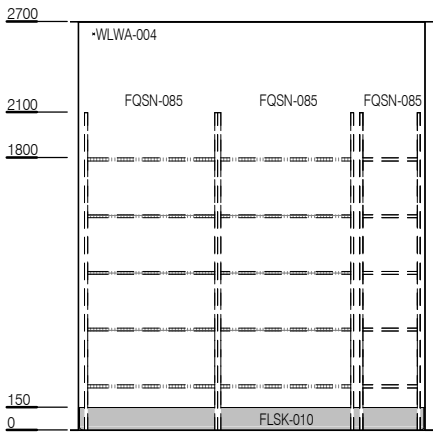
ELEVATION 2
