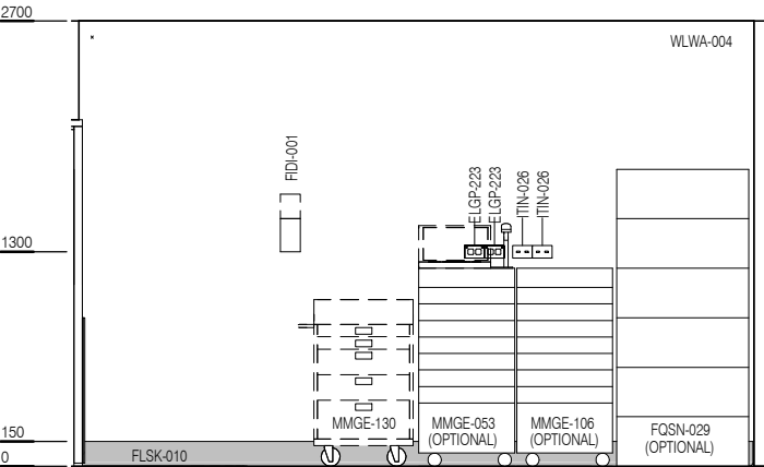
ELEVATION 4
