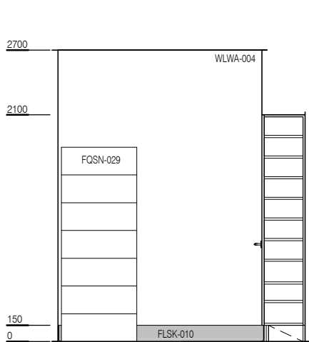
ELEVATION 1
