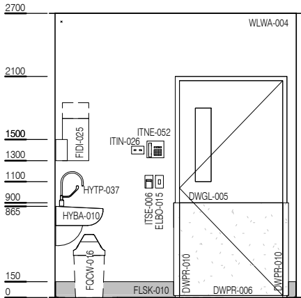
ELEVATION 3
