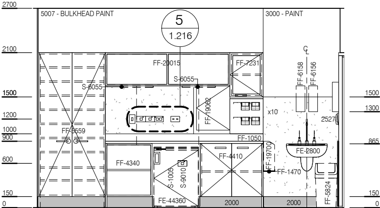
ELEVATION 2
