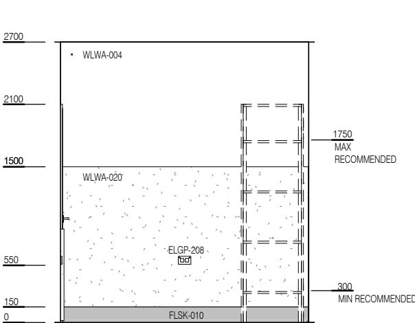
ELEVATION 4
