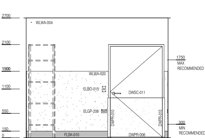
ELEVATION 3
