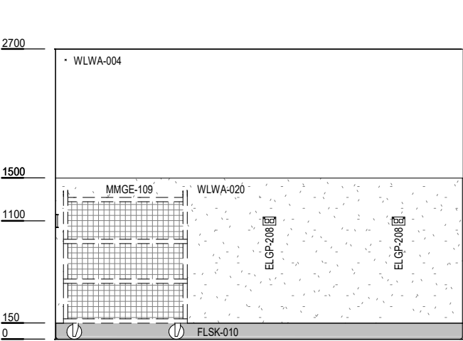
ELEVATION 4
