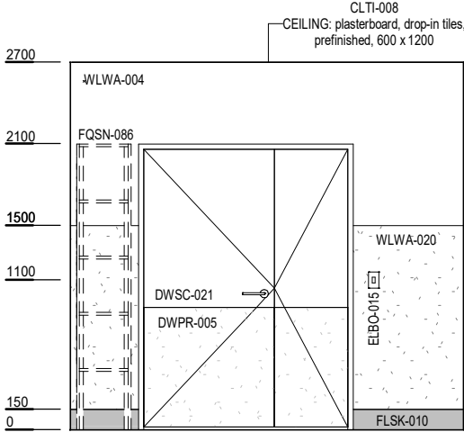
ELEVATION 3
