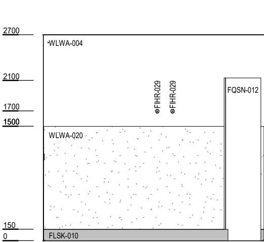
ELEVATION 1
