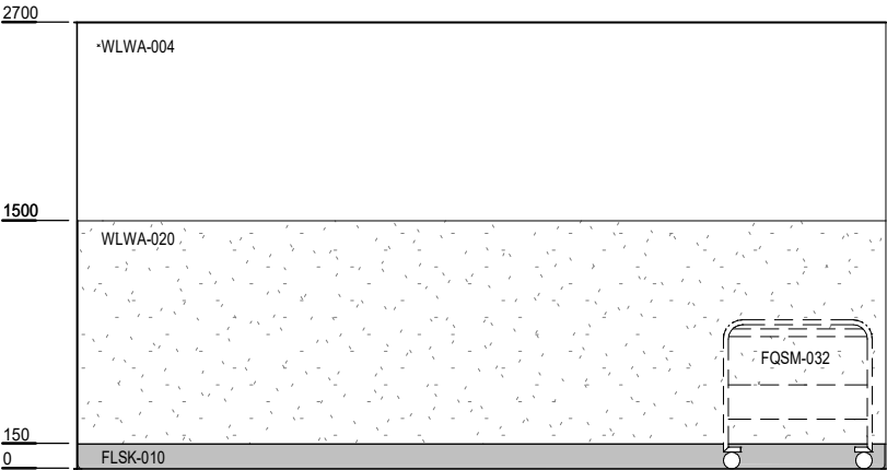
ELEVATION 4
