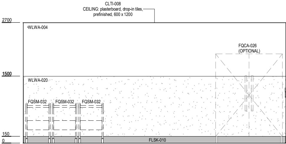
ELEVATION 1
