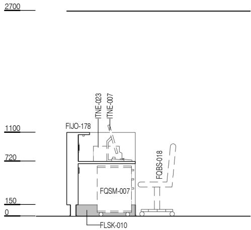
ELEVATION 1
