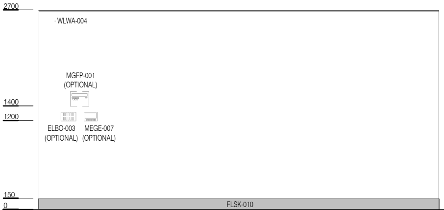
ELEVATION 2
