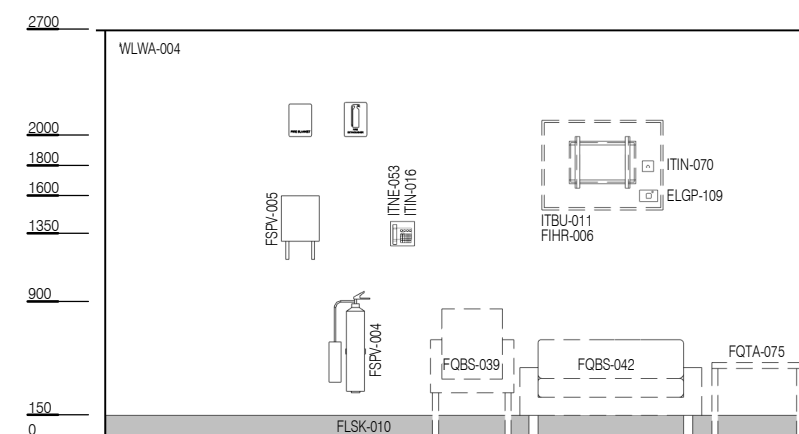
ELEVATION 4
