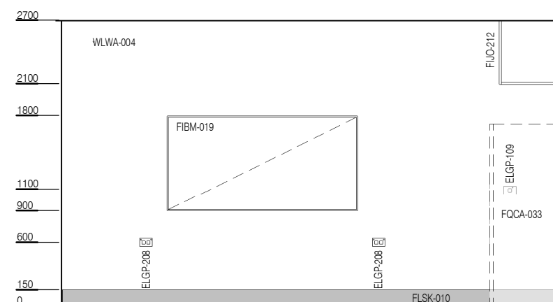
ELEVATION 2
