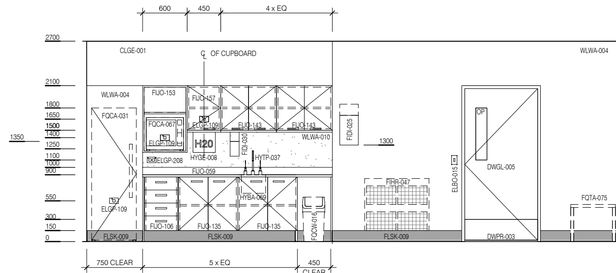
ELEVATION 3
