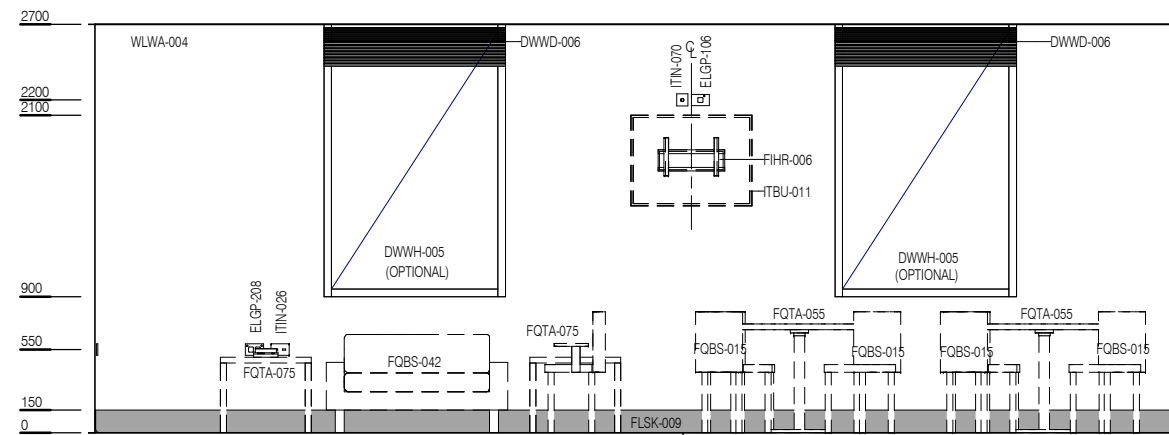
ELEVATION 1
