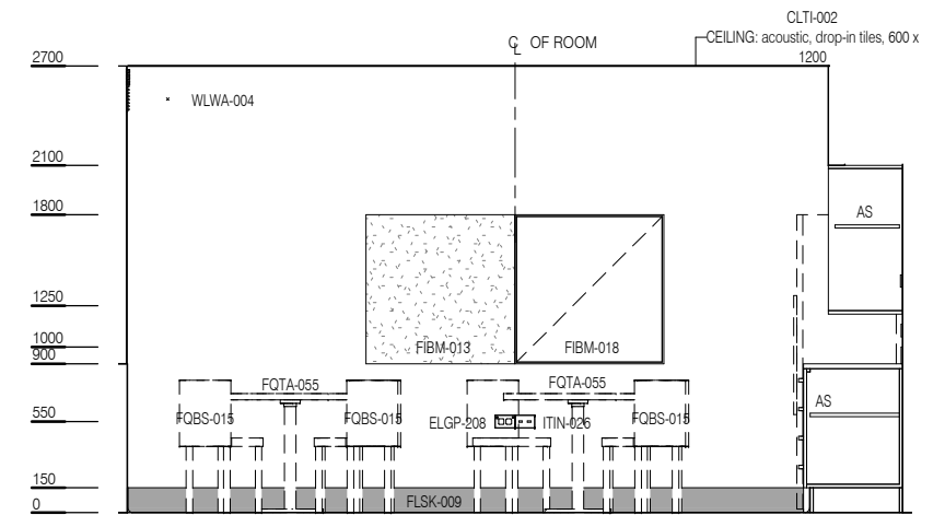
ELEVATION 2
