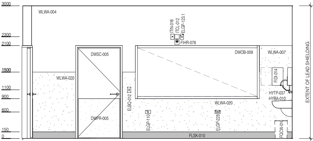
ELEVATION 3
