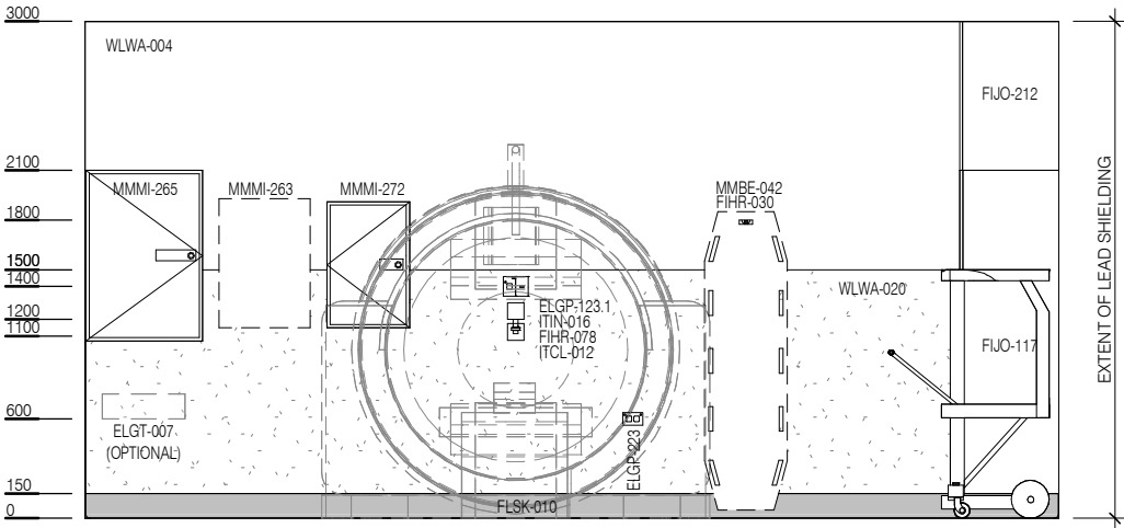
ELEVATION 1
