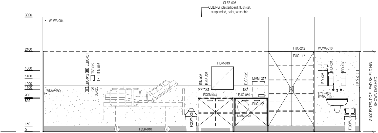
ELEVATION 4
