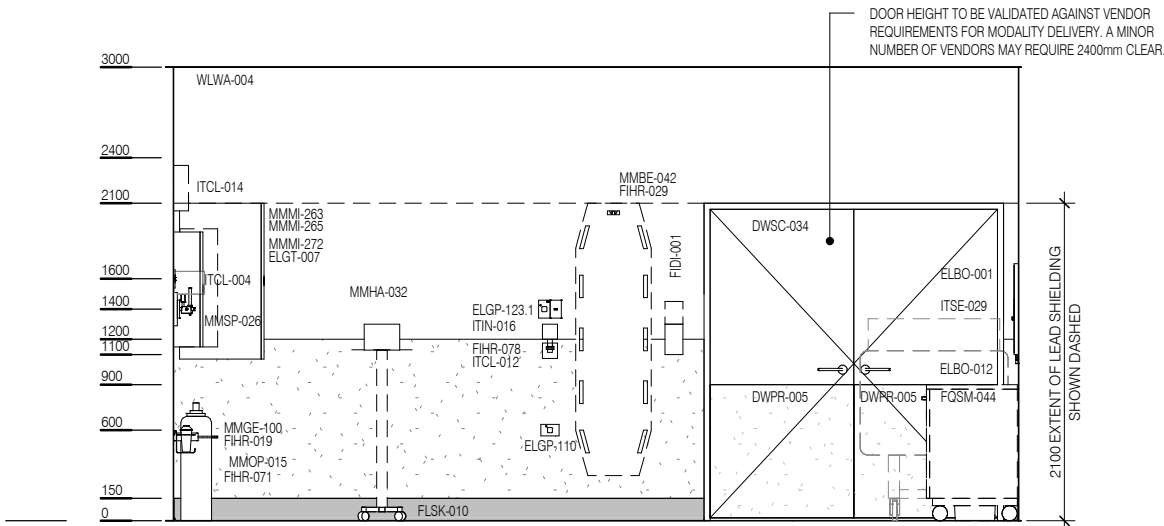
ELEVATION 3
