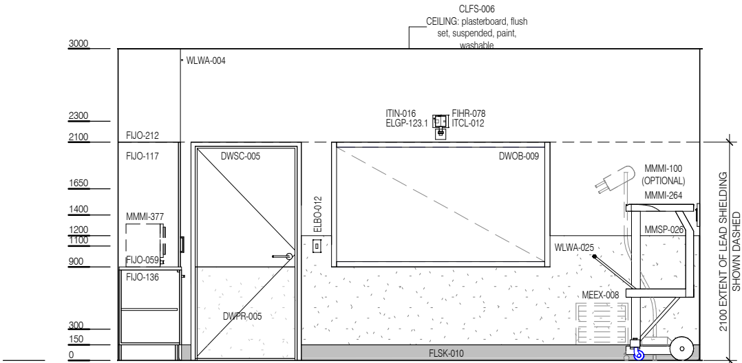
ELEVATION 1
