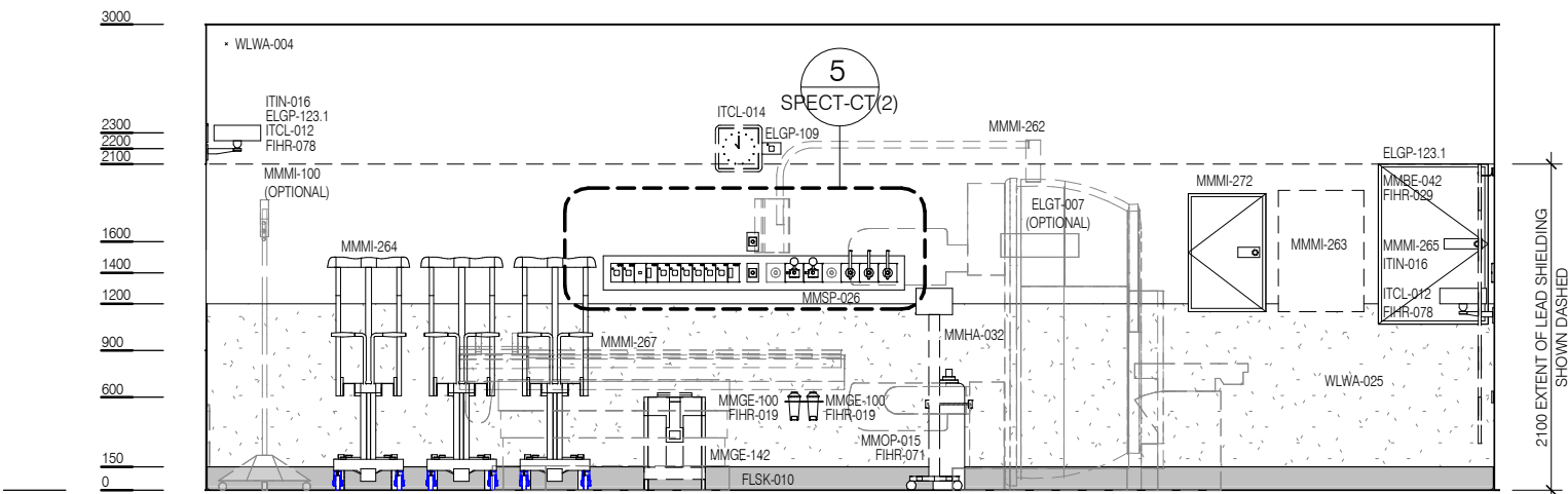
ELEVATION 2
