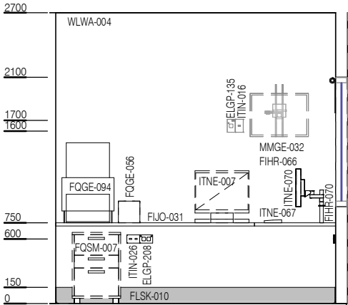
ELEVATION 2
