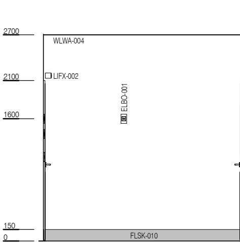
ELEVATION 4
