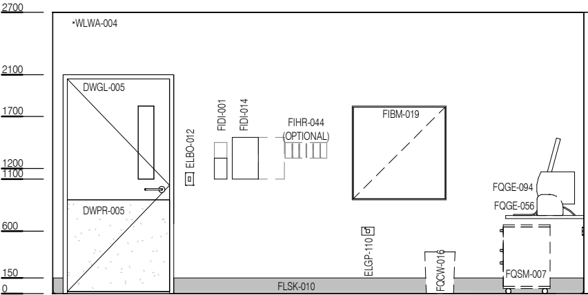
ELEVATION 1
