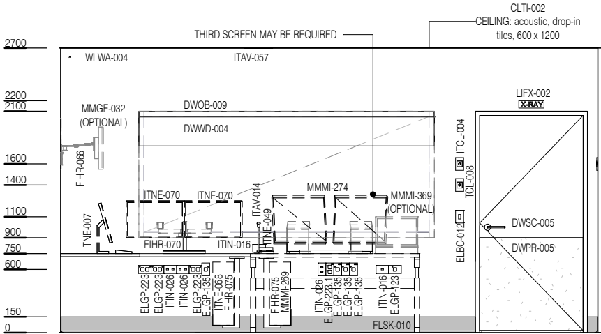
ELEVATION 3
