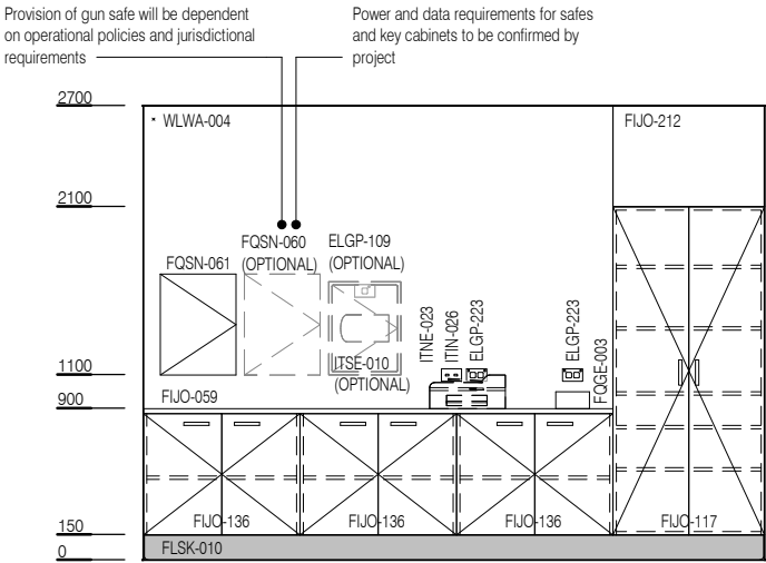
ELEVATION 4
