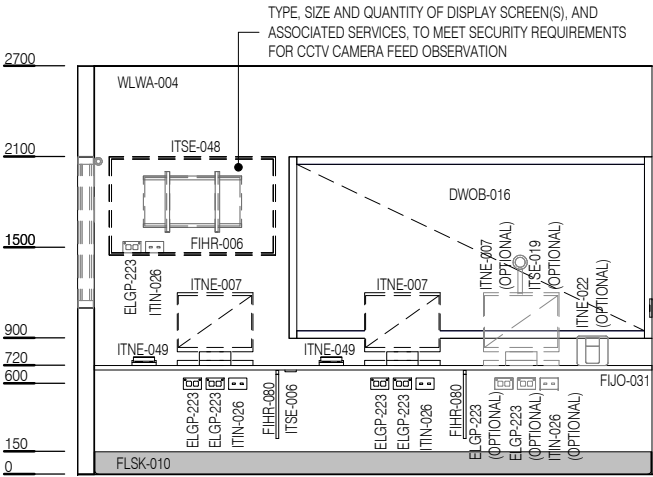
ELEVATION 2
