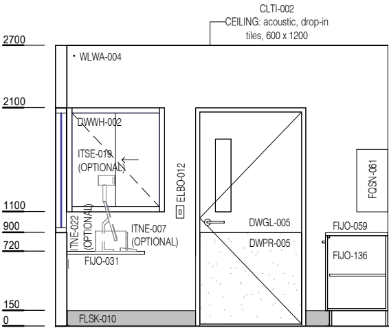
ELEVATION 3
