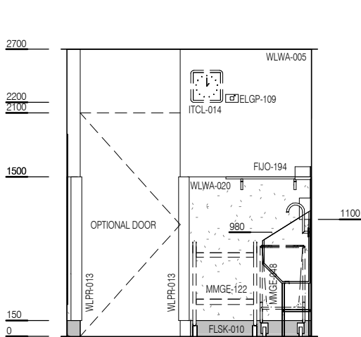
ELEVATION 3
