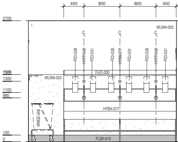
ELEVATION 4
