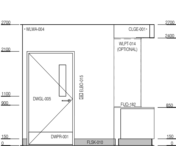
ELEVATION 3
