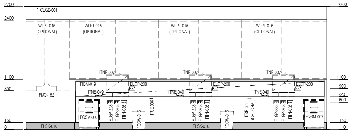
ELEVATION 4
