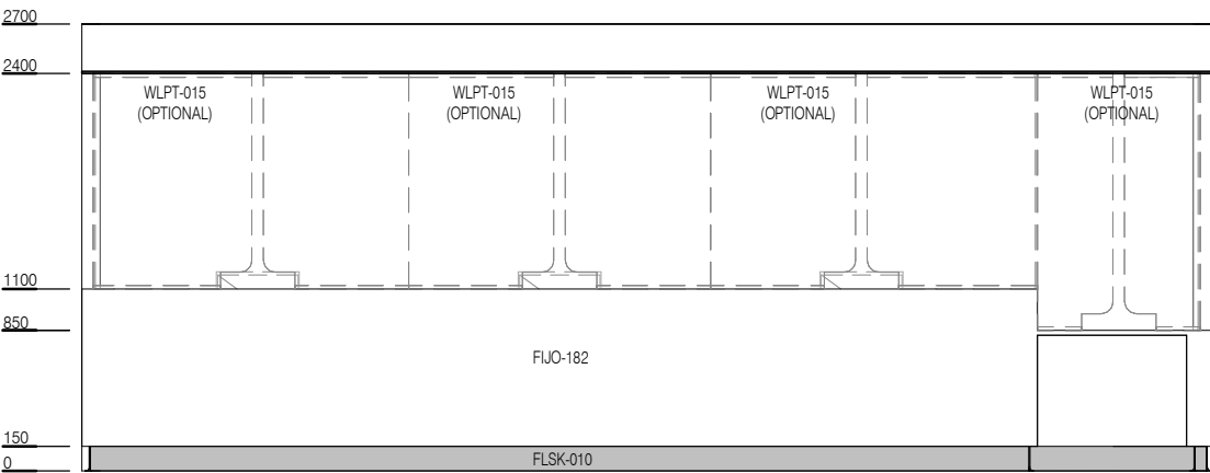
ELEVATION 5
