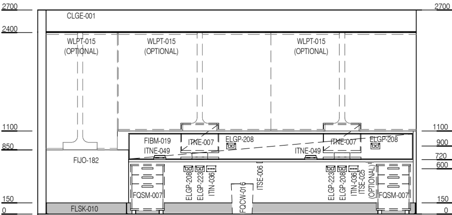
ELEVATION 4
