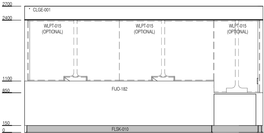
ELEVATION 5
