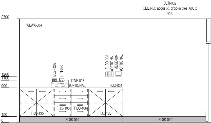
ELEVATION 2
