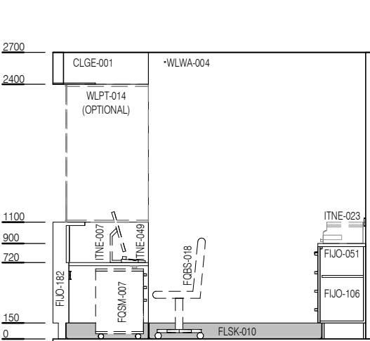
ELEVATION 1
