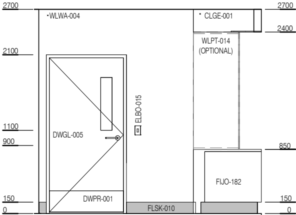
ELEVATION 3
