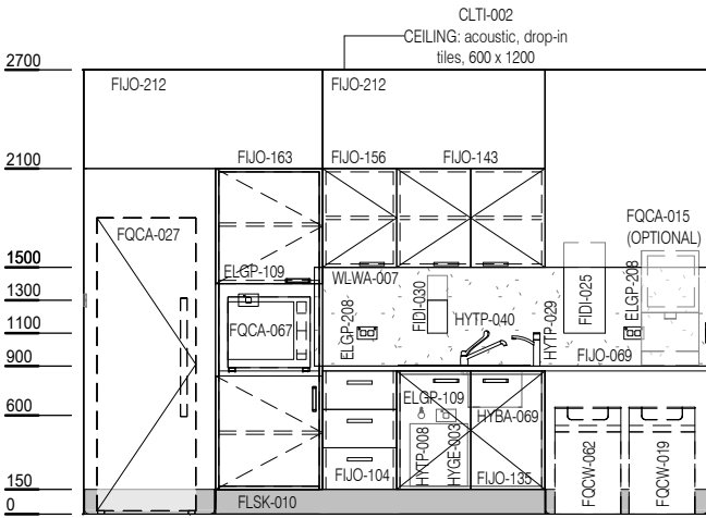
ELEVATION 2
