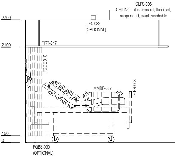
ELEVATION 2
