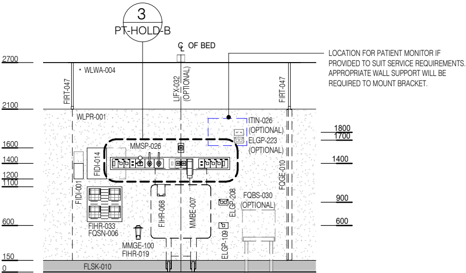
ELEVATION 1
