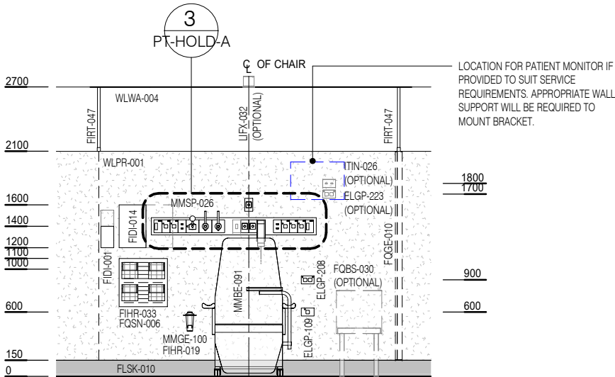
ELEVATION 1
