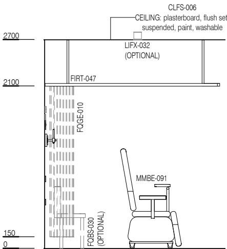
ELEVATION 2
