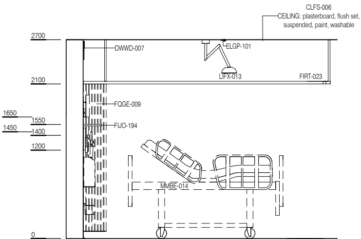
ELEVATION 2
