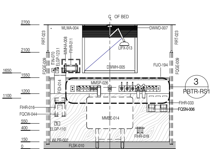
ELEVATION 1
