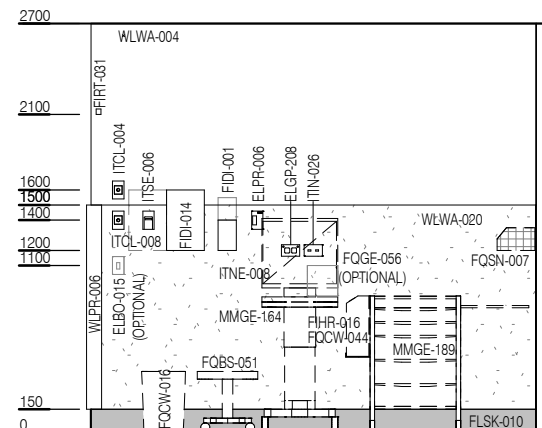
ELEVATION 1
