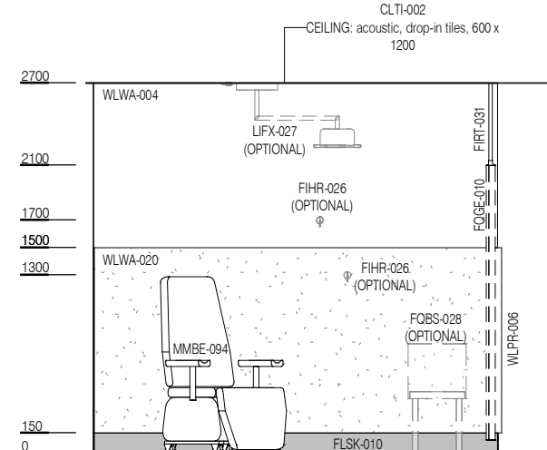
ELEVATION 3
