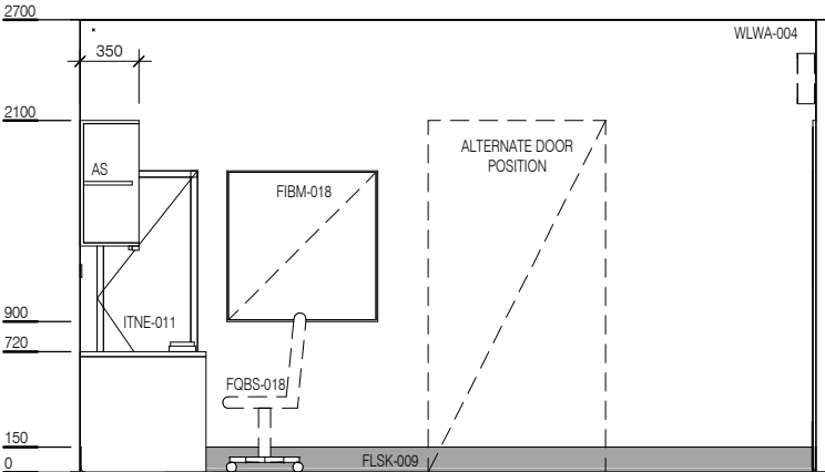
ELEVATION 2
