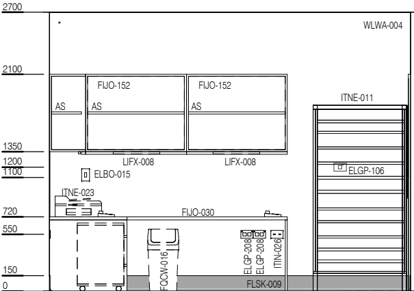
ELEVATION 1
