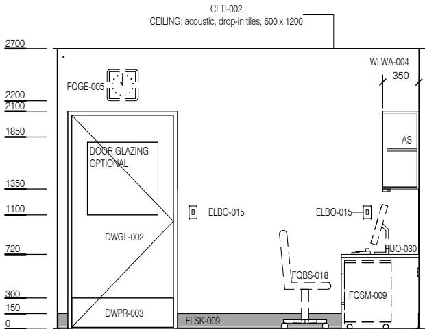
ELEVATION 3
