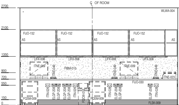
ELEVATION 4
