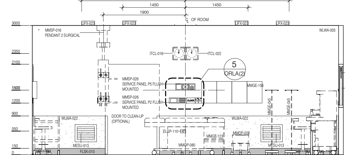
ELEVATION 4
