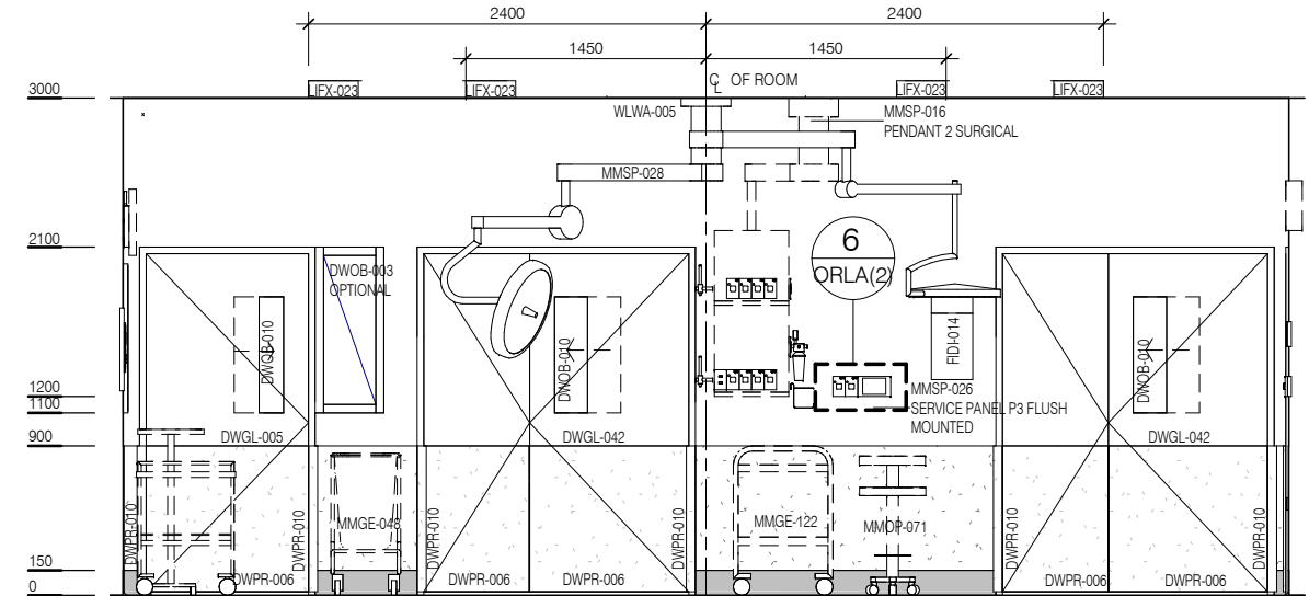
ELEVATION 3
