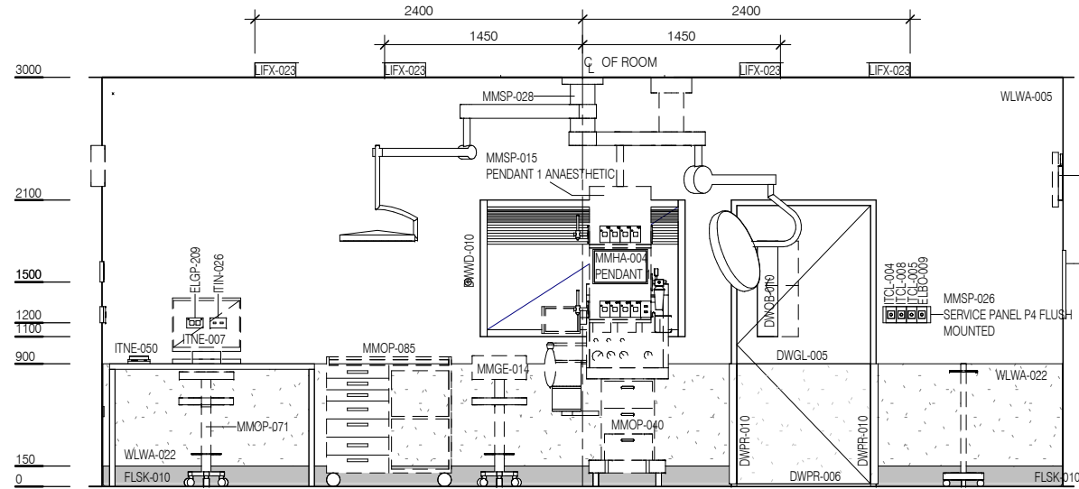
ELEVATION 1
