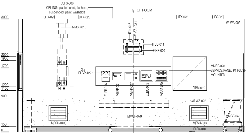
ELEVATION 2
