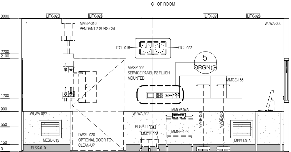
ELEVATION 2
