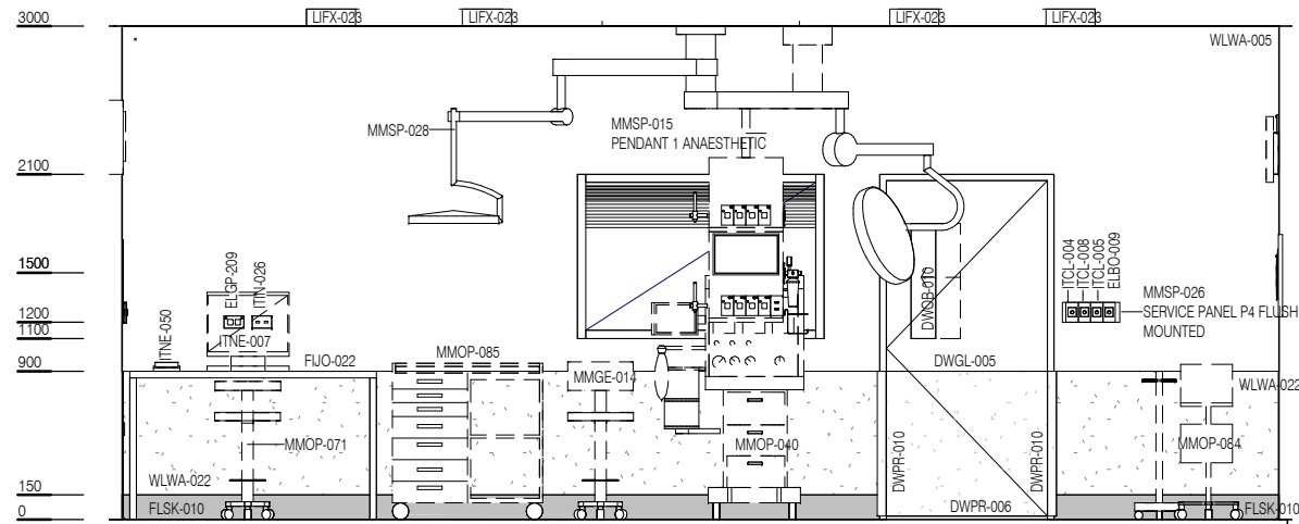
ELEVATION 1
