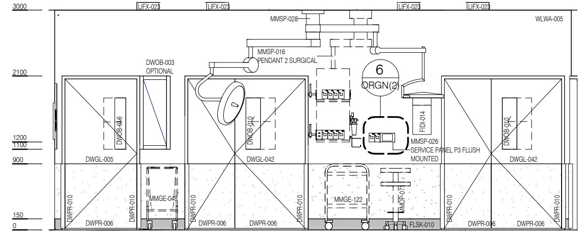
ELEVATION 3
