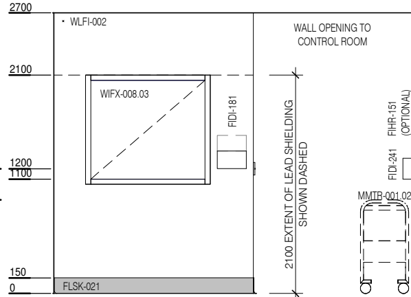
ELEVATION 3
