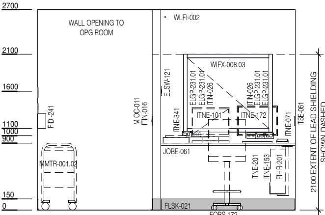
ELEVATION 5
