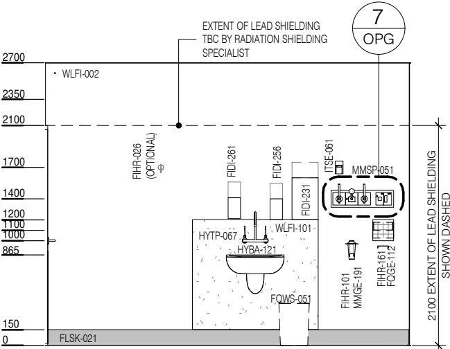
ELEVATION 1
