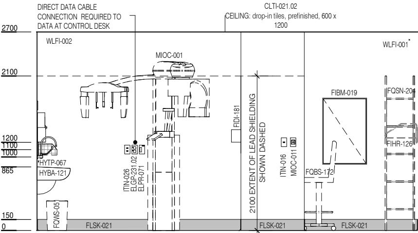
ELEVATION 2
