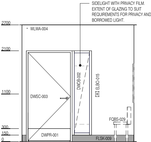
ELEVATION 3
