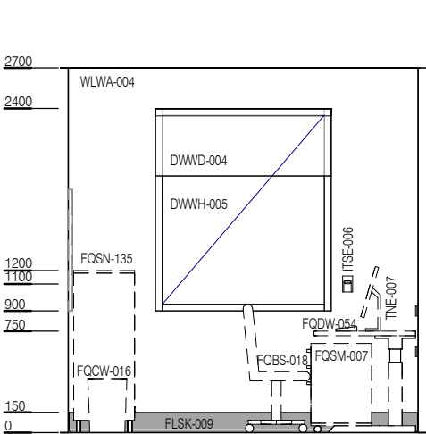
ELEVATION 1
