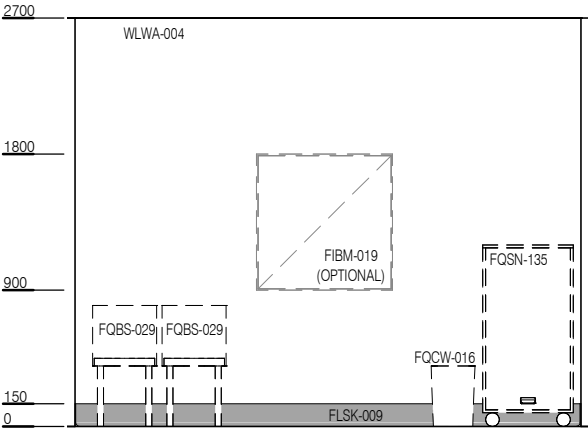
ELEVATION 4
