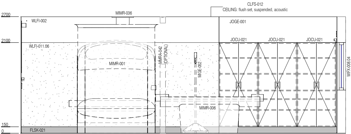
ELEVATION 2
