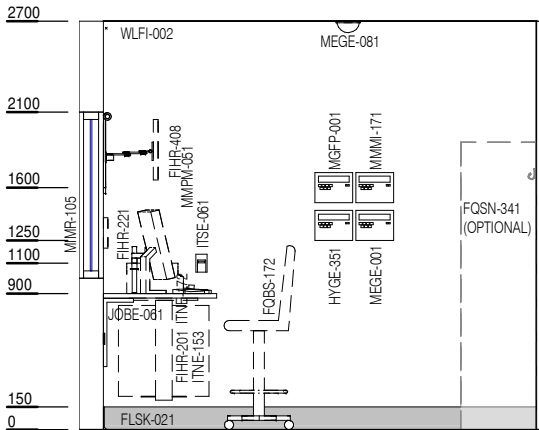
ELEVATION 2
