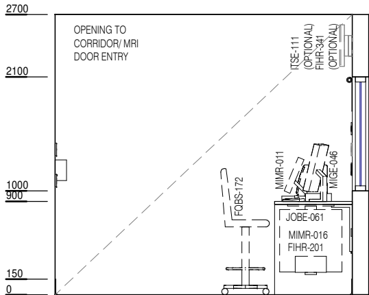
ELEVATION 4
