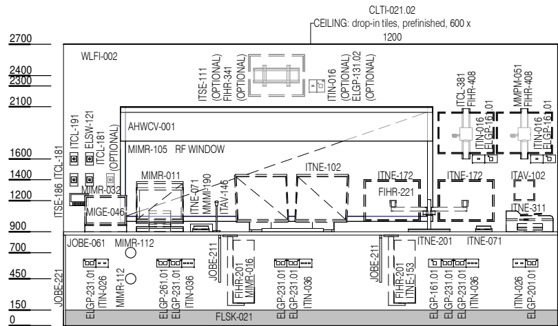
ELEVATION 1
