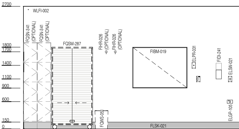
ELEVATION 3
