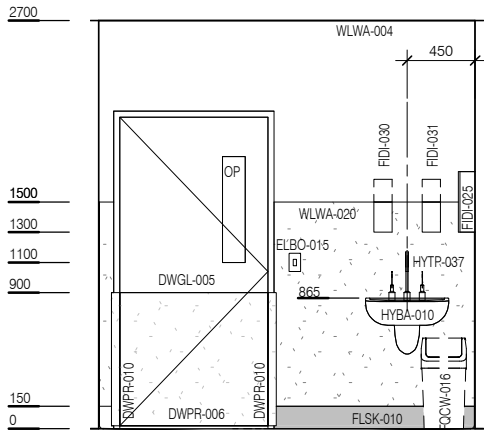
ELEVATION 3
