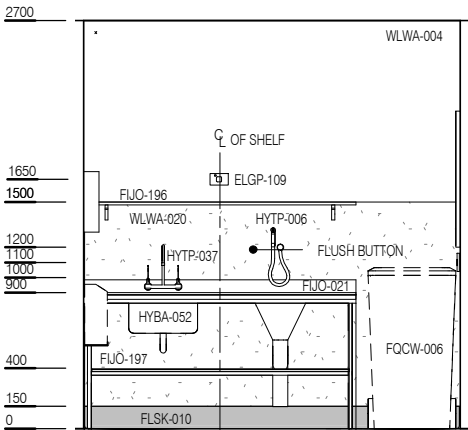
ELEVATION 1
