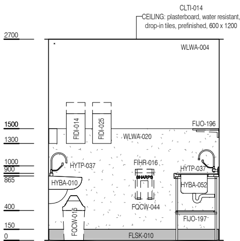
ELEVATION 4
