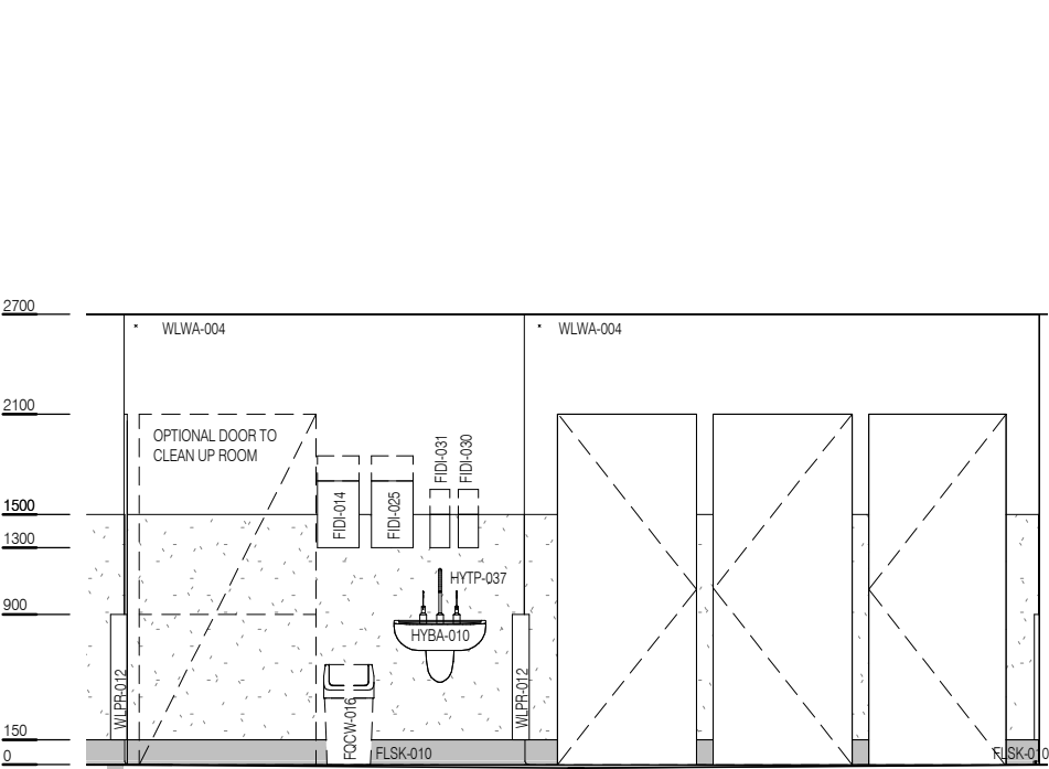
ELEVATION 2
