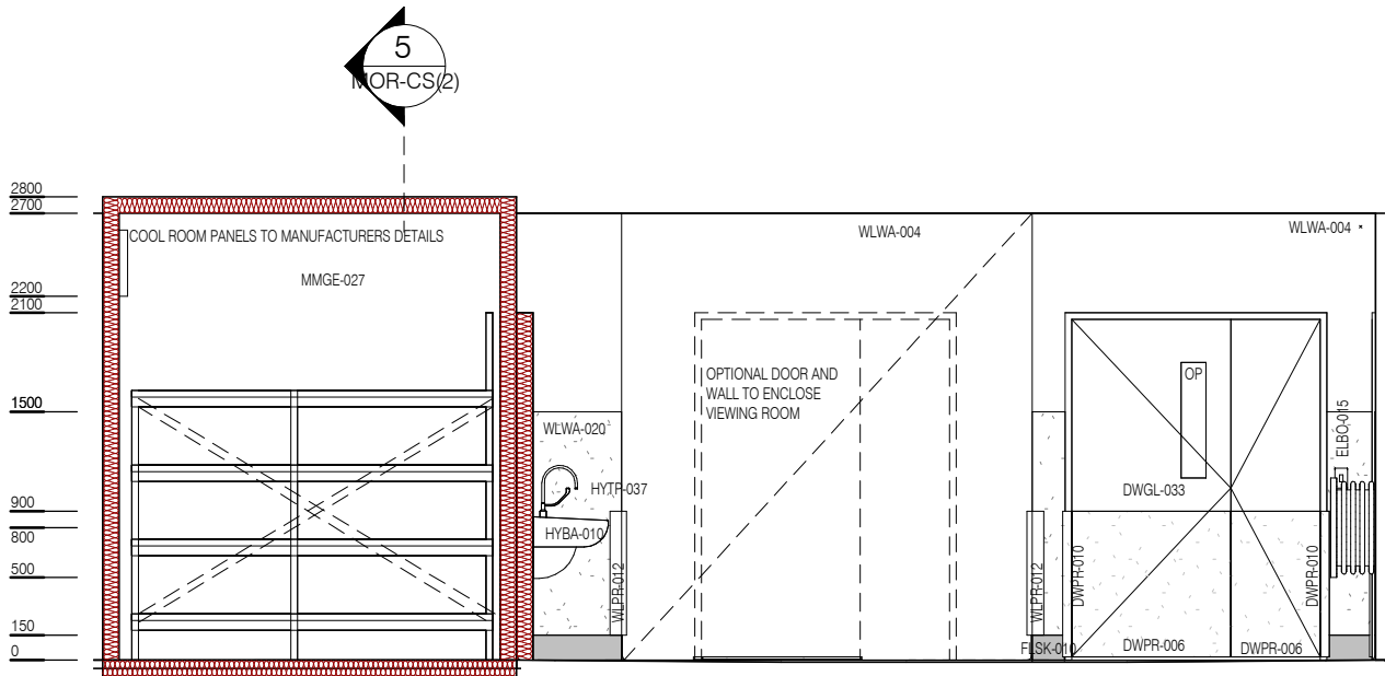
ELEVATION 1
