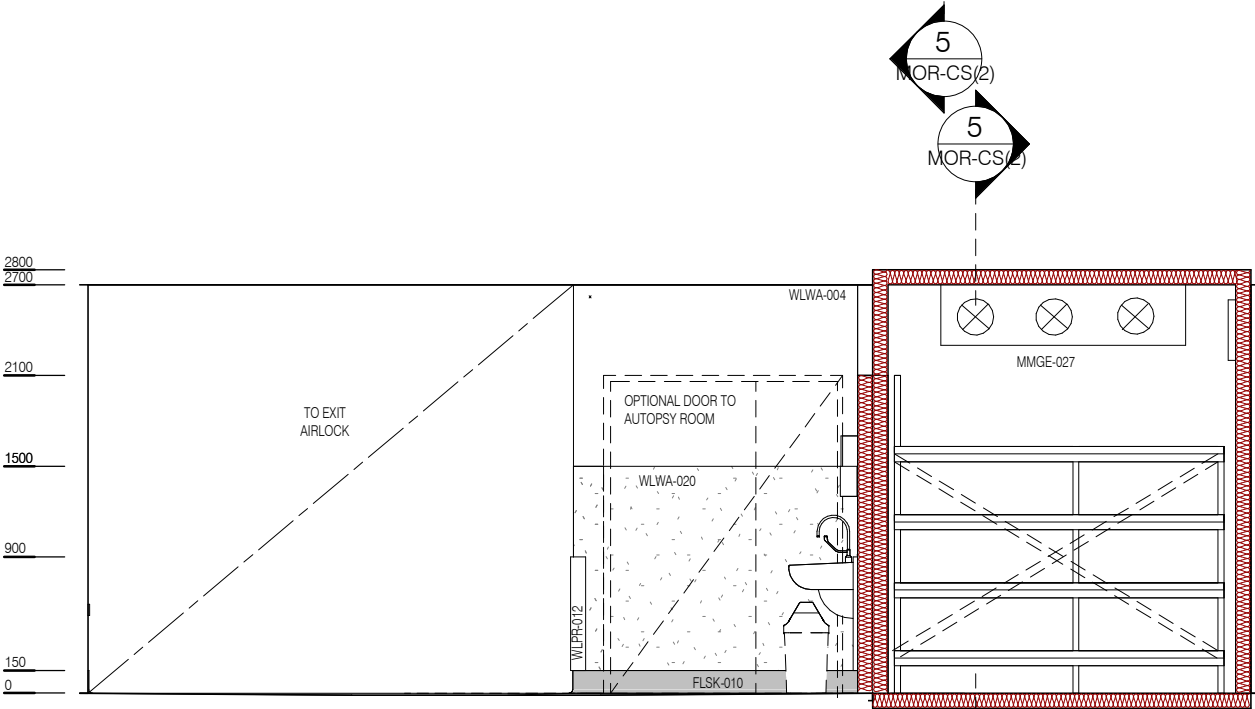
ELEVATION 1
