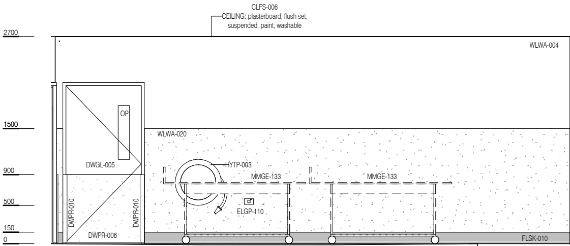
ELEVATION 2
