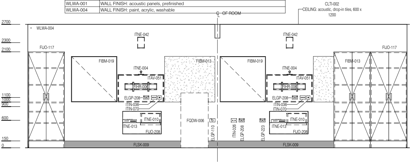
ELEVATION 1
