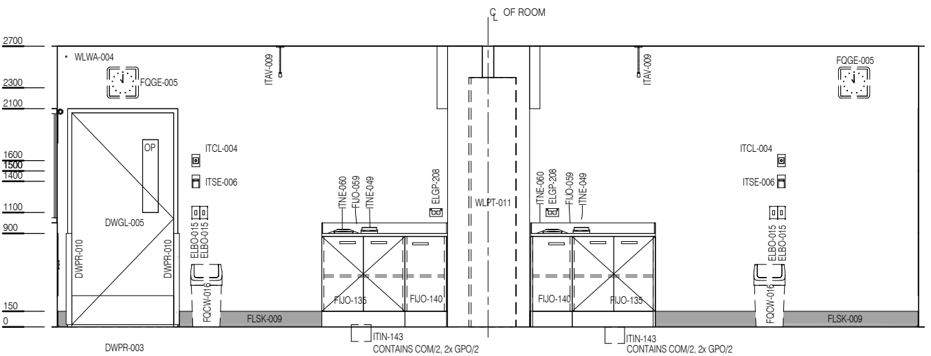
ELEVATION 3
