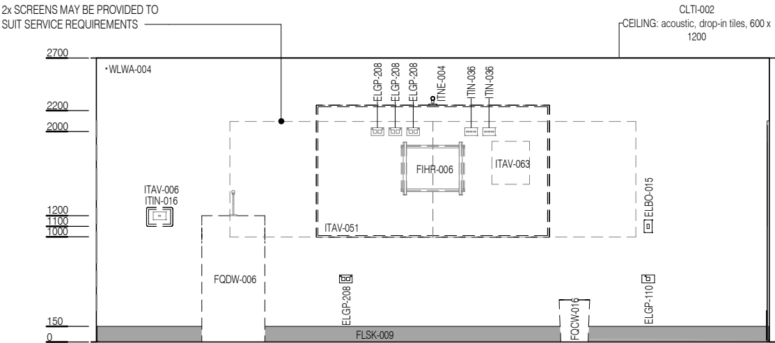
ELEVATION 1
