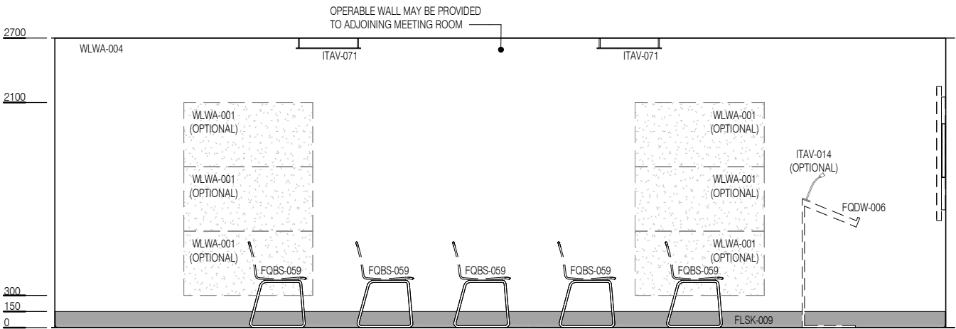
ELEVATION 4
