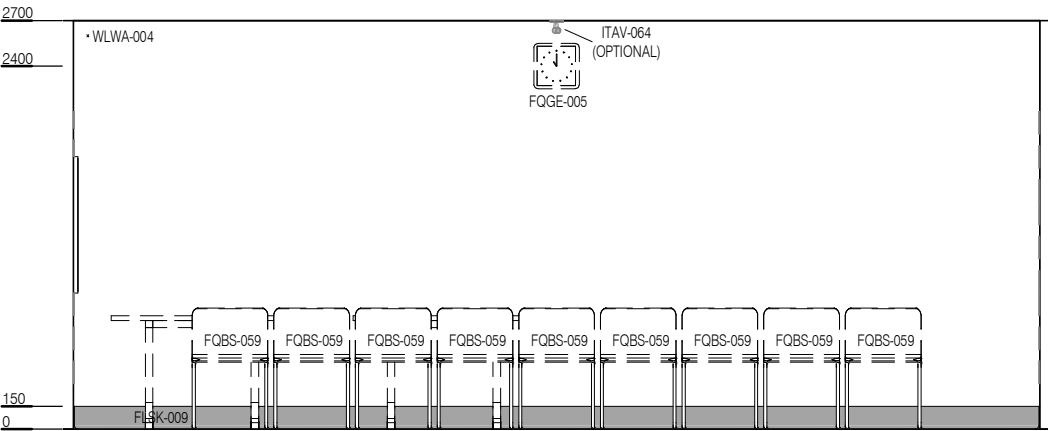
ELEVATION 3
