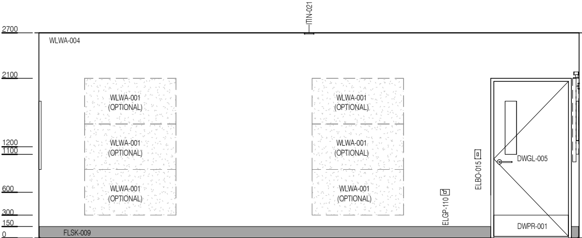
ELEVATION 4
