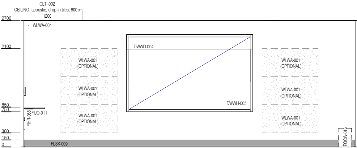
ELEVATION 2
