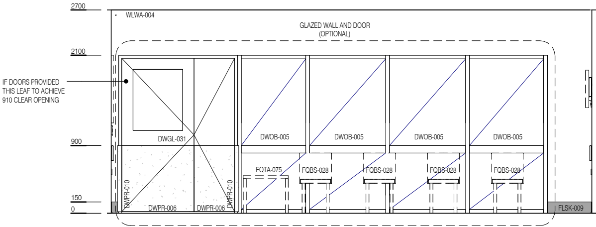
ELEVATION 3
