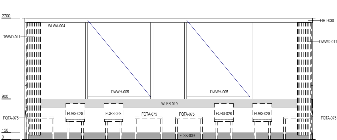
ELEVATION 1
